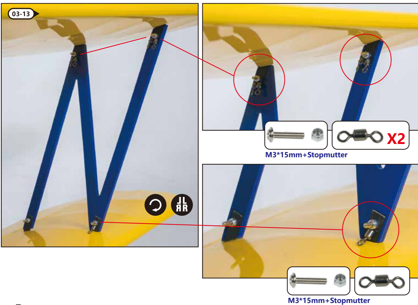
Tragflächen in den Rumpf einsetzen und festschrauben.
