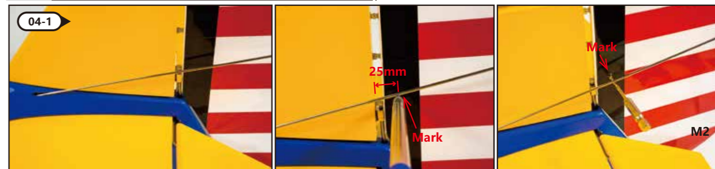
Anlenkungsdraht in den Rumpf einführen und die Anschlussstelle am Ruderhorn markieren, anschließend bohren.
