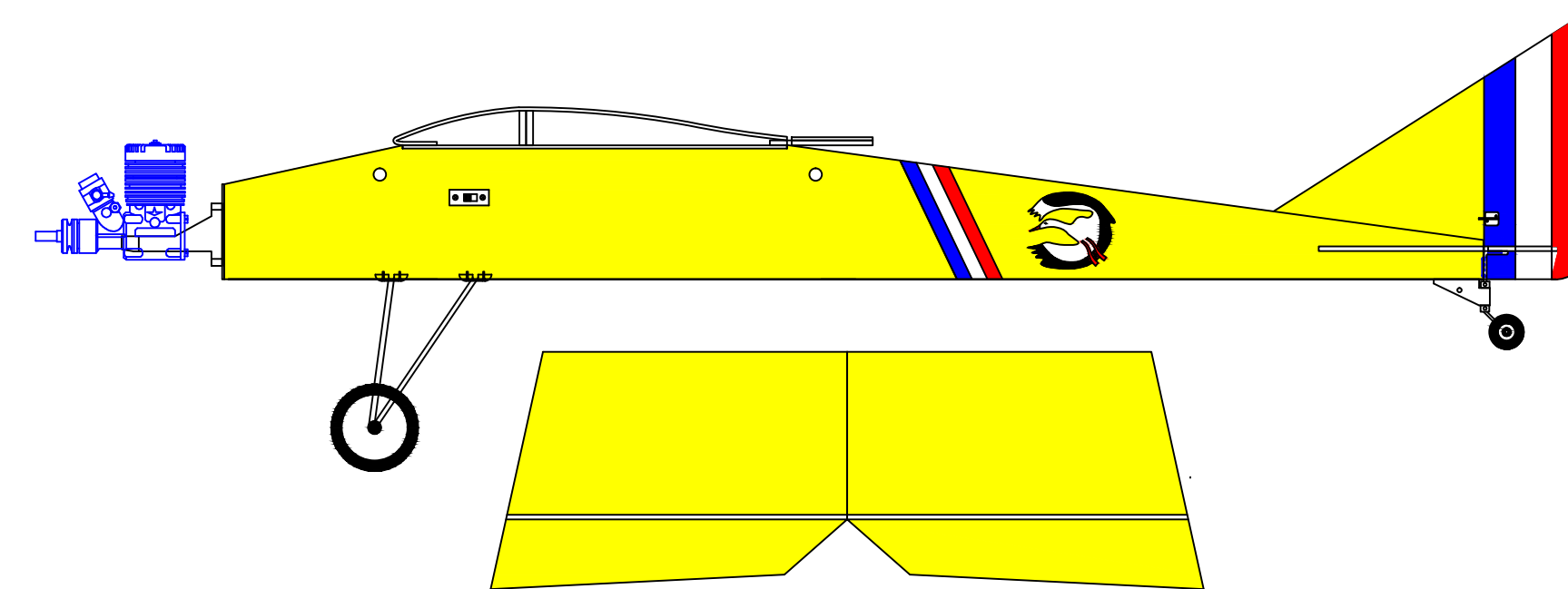
PIANI DI CODA "TIPO FRANCESE"
