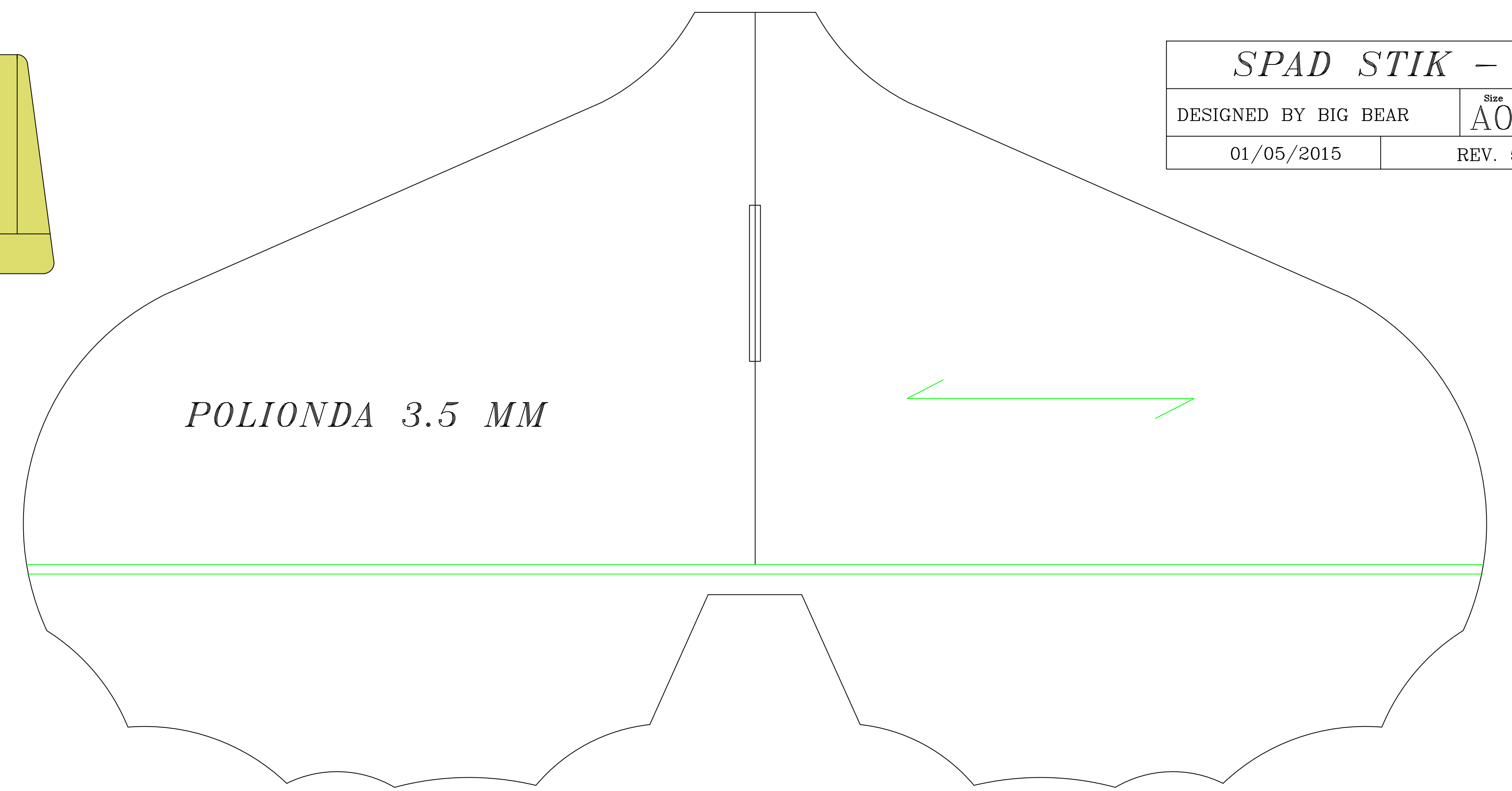
PIANI DI CODA "TIPO ITALIANO"
