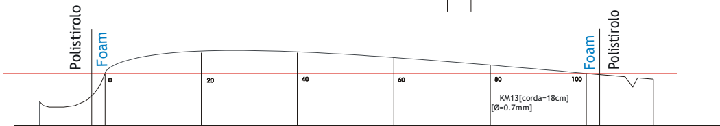
Dima per taglio estradosso Upper profile template
