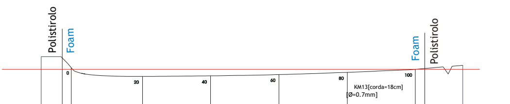
Dima per taglio intradosso Lower profile template
