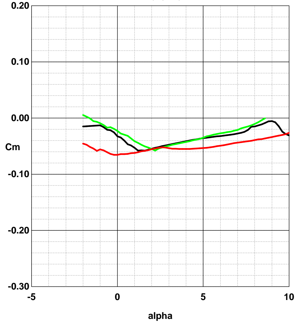
Cm(alpha):
