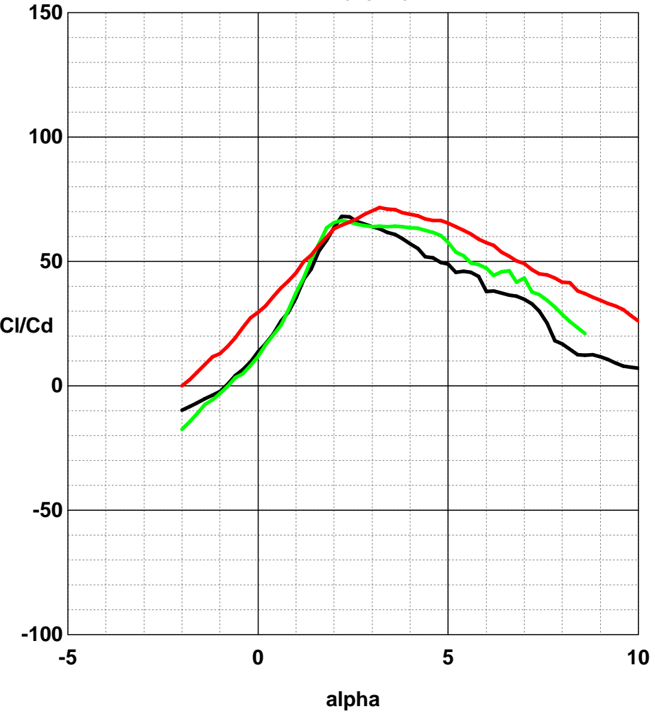
Cl/Cd(alpha):
