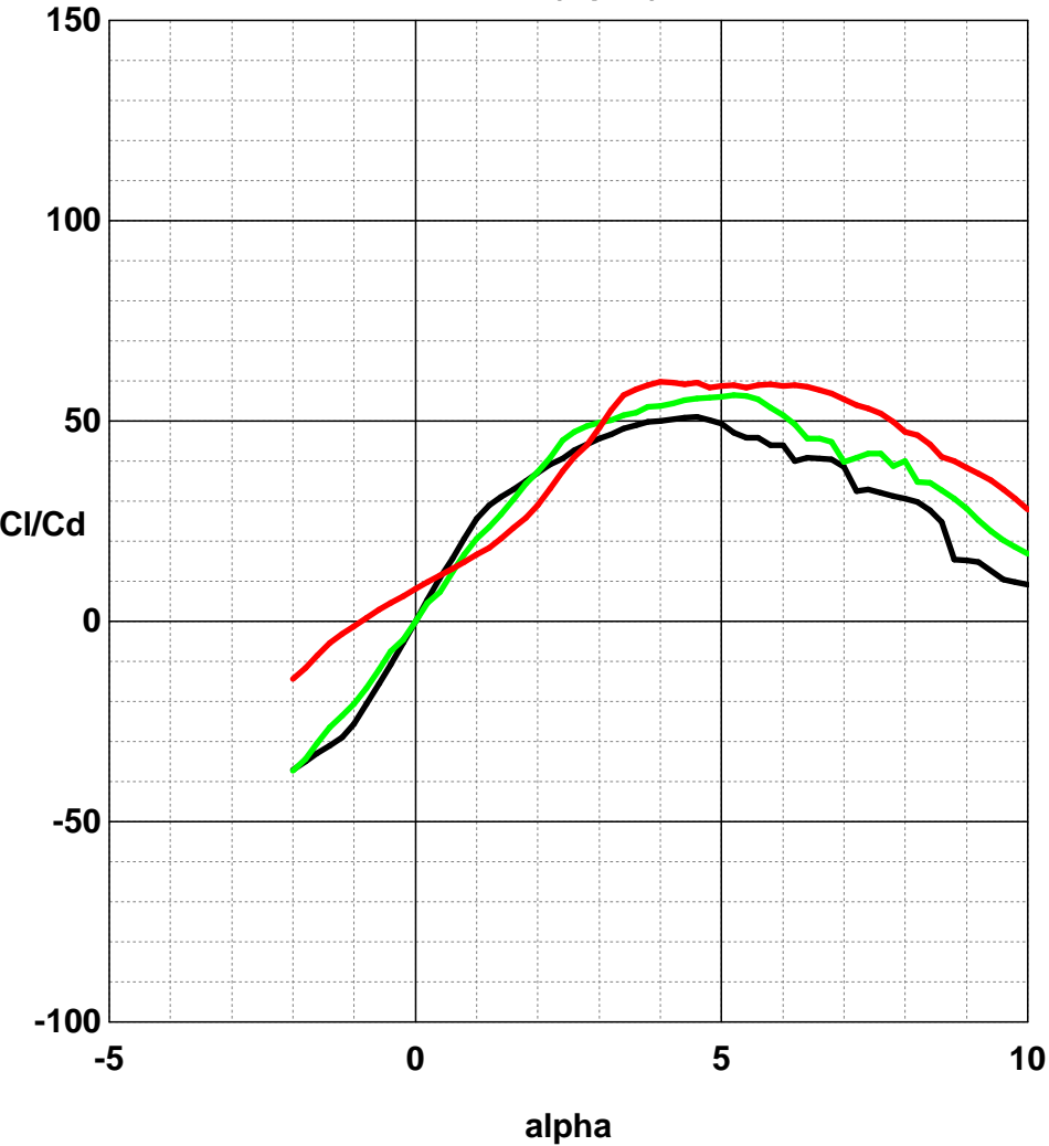
Cl/Cd(alpha):
