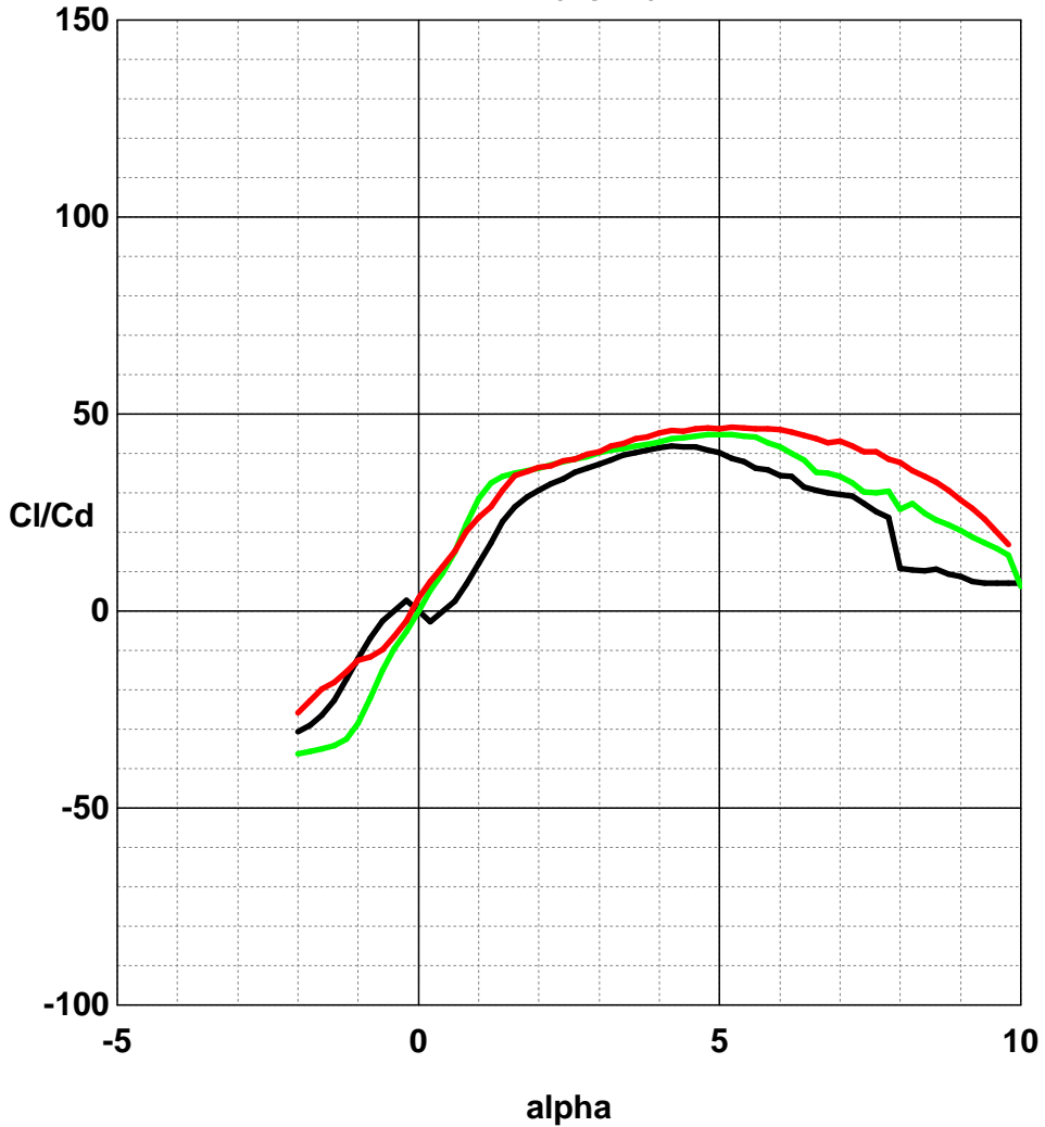
Cl/Cd(alpha):
