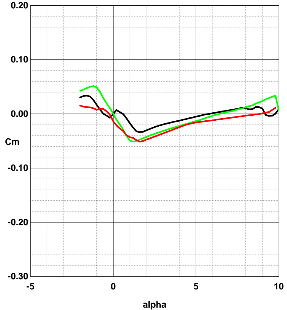
Cm(alpha):
