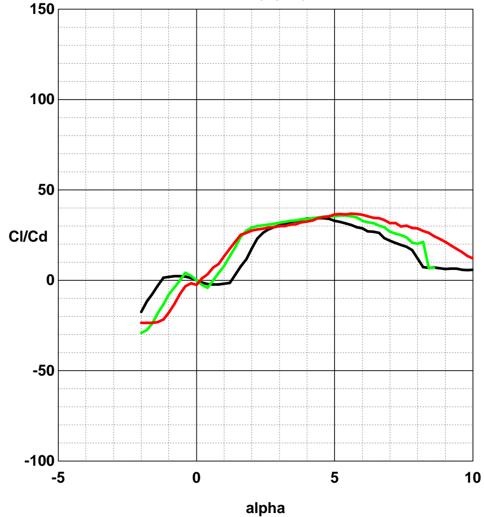
Cl/Cd(alpha):
